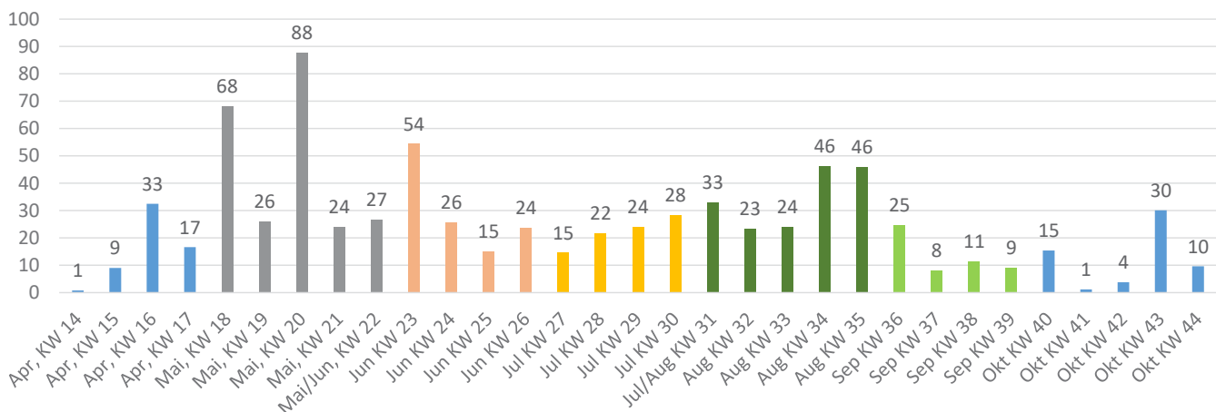
Regen in mm (Wochensummen) 2018, Wetterstation „Pöbnitz Süd“
