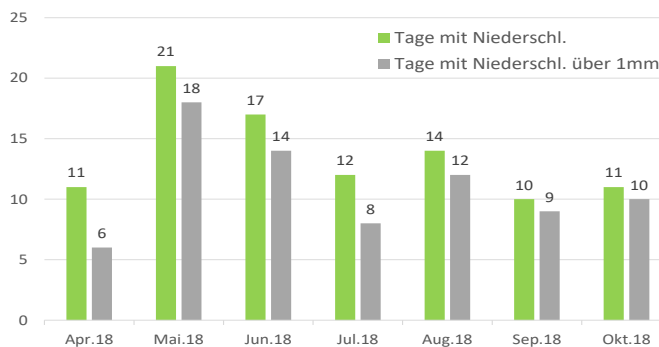
Anzahl der Tage mit gemessenen Niederschlägen, Wetterstation „Pöbnitz Süd“, 2018
