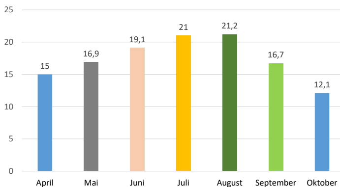
Temperatur °C: Monatsmittelwerte 2018, Wetterstation „Pöbnitz Süd“
